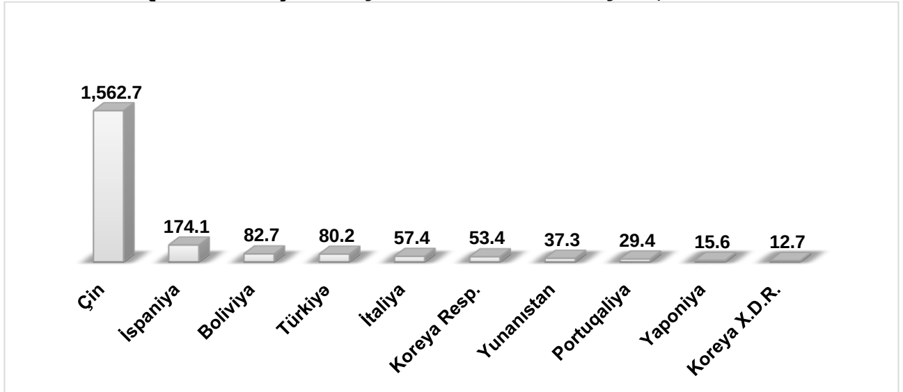
Qrafik 9. Dünya üzrə şabalıdın əsas istehsalçıları, min ton
