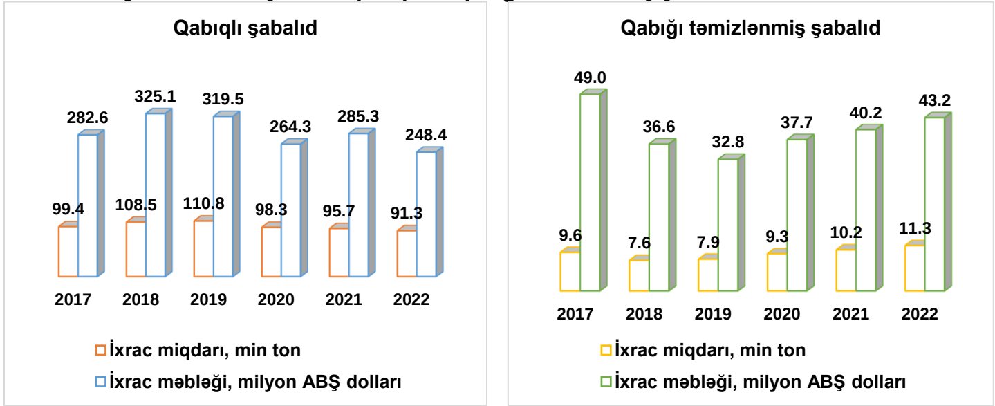
Qrafik 10. Dünya üzrə qabıqlı və qabığı təmizlənmiş şabalıd ixracının həcmi
