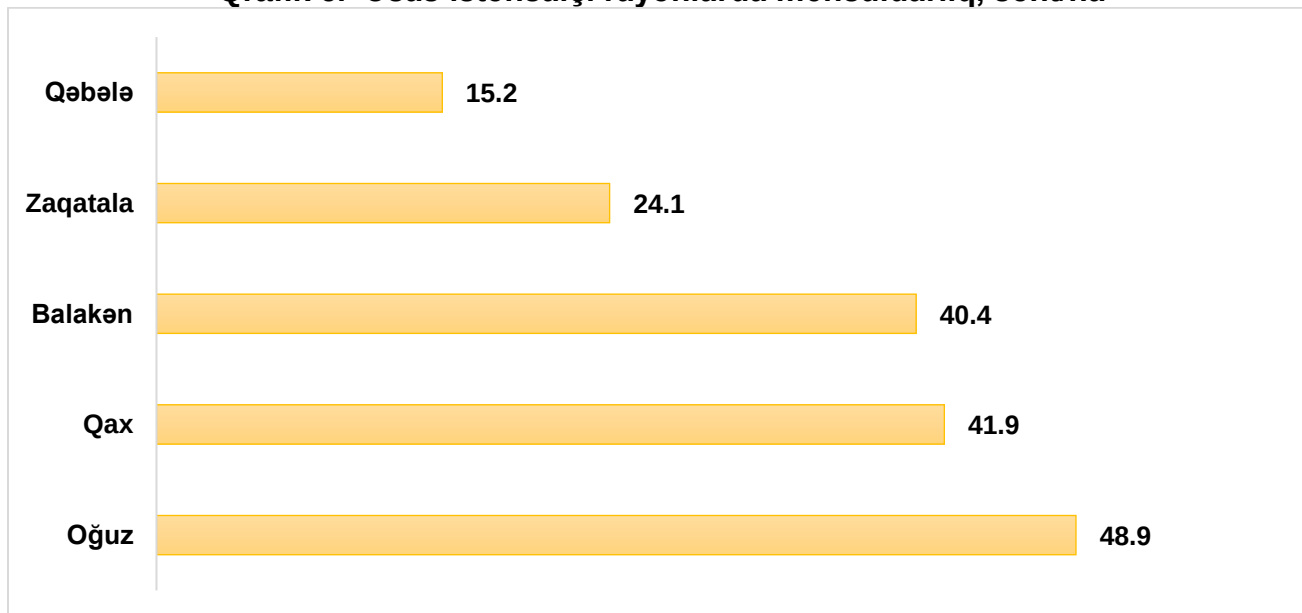
Qrafik 6. Əsas istehsalçı rayonlarda məhsuldarlıq, sent/ha
