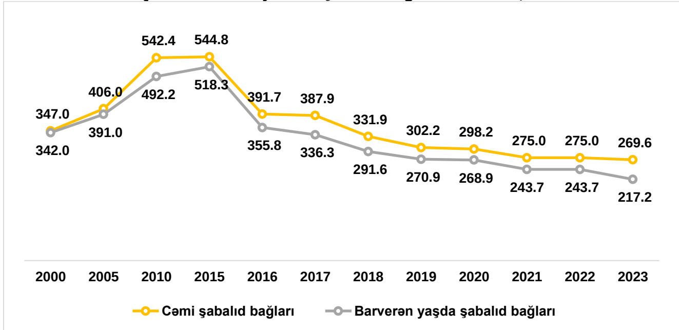
Qrafik 1. Azərbaycanda şabalıd bağlarının sahəsi, ha
