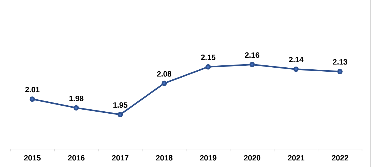
Qrafik 8. Şabalıdın qlobal istehsal göstəriciləri, milyon ton
