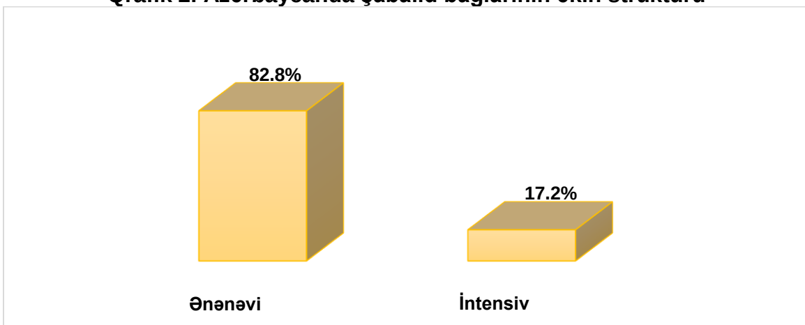
Qrafik 2. Azərbaycanda şabalıd bağlarının əkin strukturu
