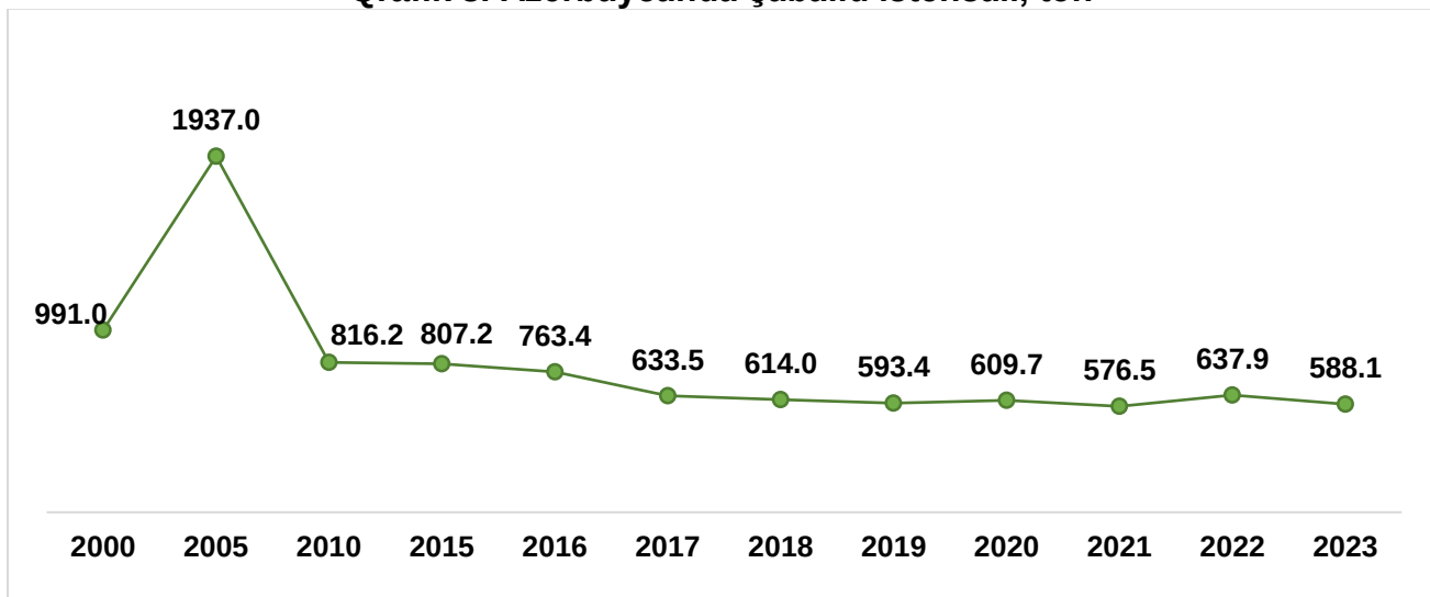
Qrafik 3. Azərbaycanda şabalıd istehsalı, ton
