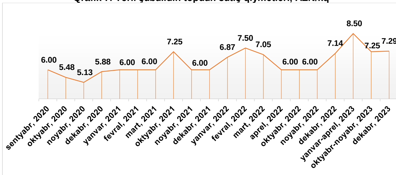
Qrafik 7. Yerli şabalıdın topdan satış qiymətləri, AZN/kq
