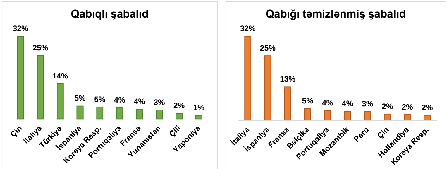
Qrafik 11. Qlobal bazarda qabıqlı və qabığı təmizlənmiş şabalıd ixracının ölkələr üzrə strukturu
