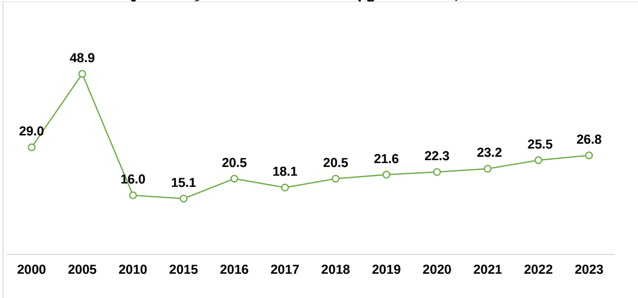
Qrafik 5. Şabalıdın məhsuldarlıq göstəriciləri, sent/ha
