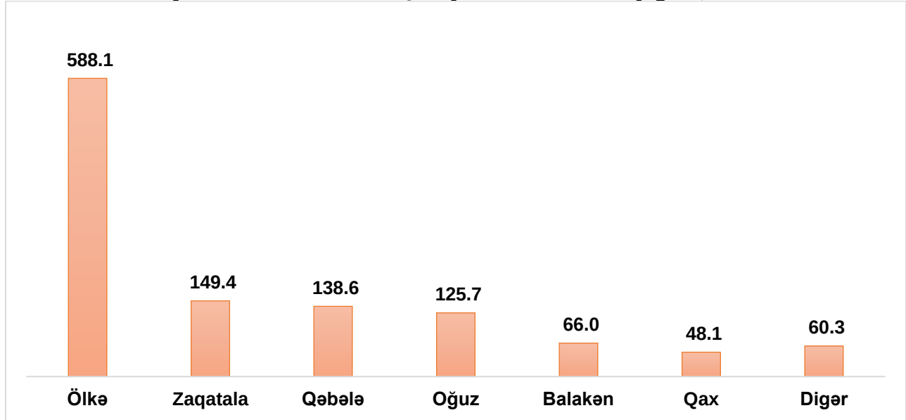
Qrafik 4. Əsas istehsalçı rayonlarda məhsul yığımı, ton
